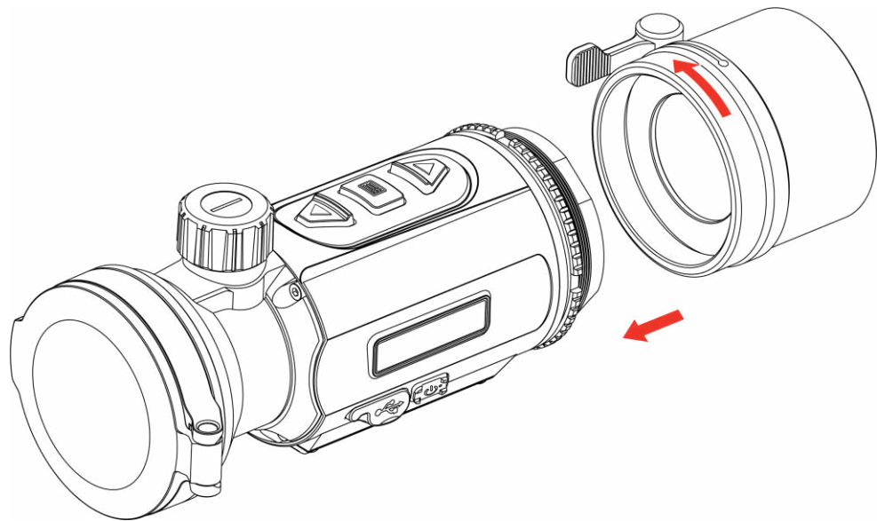
Abbildung 2-6 Adapter montieren
